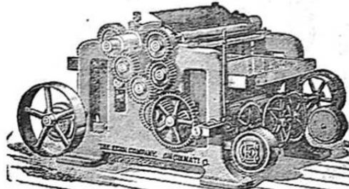
Cepillo y alisador reforzado n° 4.
